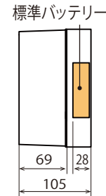
SA350 側面図
